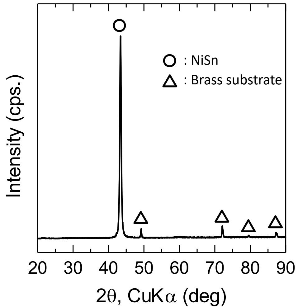
図2 Sn-Ni合金めっき皮膜のXRD回折パターン
