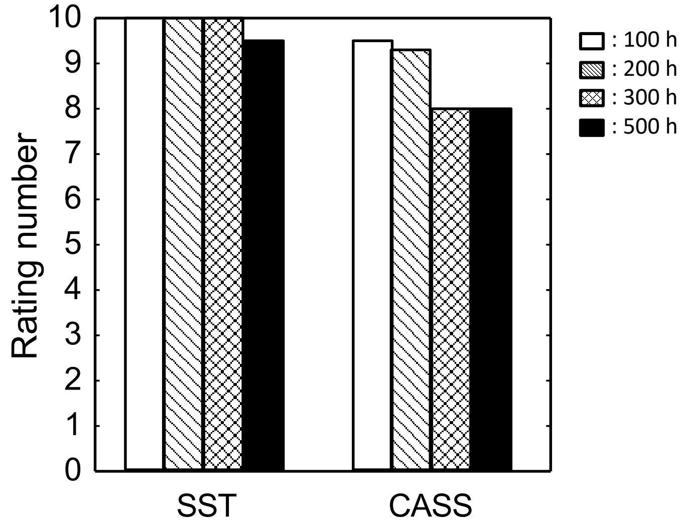
図3 Sn-Ni合金めっき皮膜の耐食性 (めっき膜厚：5 μm)
